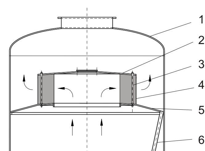
а) испаритель Роберта, б) испаритель с падающей пленкой жидкости, 1. паровая камера, 2. крышка, 3. прижимной винт крышки, 4. насадка MULTIWIR, 5. дно каплеулавливателя, 6. сливная труба.
